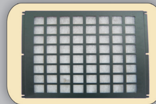
14.7217 ΦΙΛΤΡΟ ΕΞΑΕΡΙΣΜΟΥ ΚΑΜΠΙΝΑΣ Τοποθετείται στο κάτω μέρος του Rack. Περιλαμβάνει τις λαμαρινόβιδες για τη στήριξη του στο Rack (6 τεμάχια). Χρώμα RAL 9005
