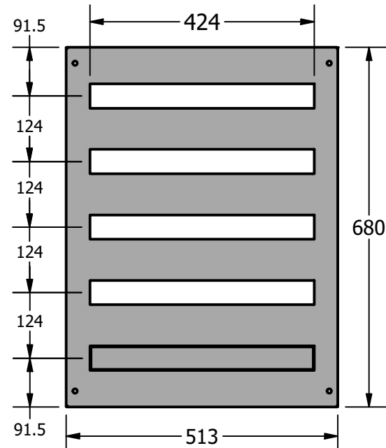
ΜΕΤΩΠΙΚΗ ΓΙΑ ΚΙΒΩΤΙΟ 55X75 5 ΣΕΙΡΩΝ-120WL
