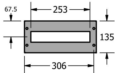
ΜΕΤΩΠΙΚΗ ΓΙΑ ΚΙΒΩΤΙΟ 35X20 1 ΣΕΙΡΑΣ-14WL
