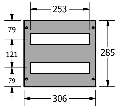
ΜΕΤΩΠΙΚΗ ΓΙΑ ΚΙΒΩΤΙΟ 35X35 2 ΣΕΙΡΩΝ-28WL
