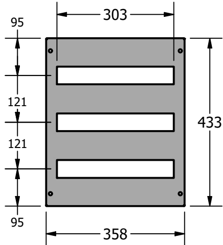
ΜΕΤΩΠΙΚΗ ΓΙΑ ΚΙΒΩΤΙΟ 40X50 3 ΣΕΙΡΩΝ-51WL
