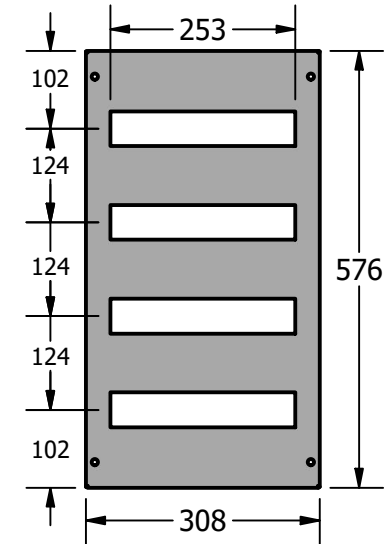
ΜΕΤΩΠΙΚΗ ΓΙΑ ΚΙΒΩΤΙΟ 35X65 4 ΣΕΙΡΩΝ-56WL
