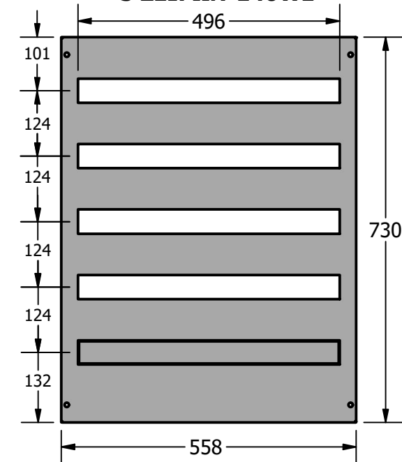
ΜΕΤΩΠΙΚΗ ΓΙΑ ΚΙΒΩΤΙΟ 60X80 5 ΣΕΙΡΩΝ-140WL
