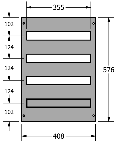
ΜΕΤΩΠΙΚΗ ΓΙΑ ΚΙΒΩΤΙΟ 45X65 4 ΣΕΙΡΩΝ-80WL
