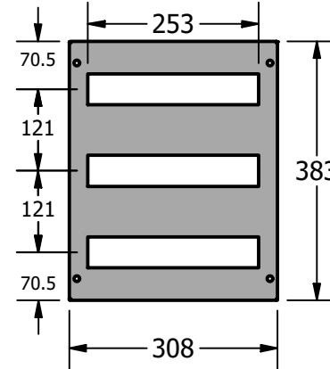
ΜΕΤΩΠΙΚΗ ΓΙΑ ΚΙΒΩΤΙΟ 35X45 3 ΣΕΙΡΩΝ-42WL
