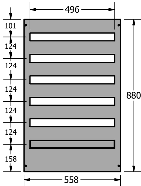
ΜΕΤΩΠΙΚΗ ΓΙΑ ΚΙΒΩΤΙΟ 60X95 6 ΣΕΙΡΩΝ
