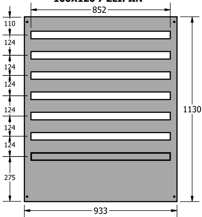
ΜΕΤΩΠΙΚΗ ΓΙΑ ΚΙΒΩΤΙΟ 100X120 7 ΣΕΙΡΩΝ
