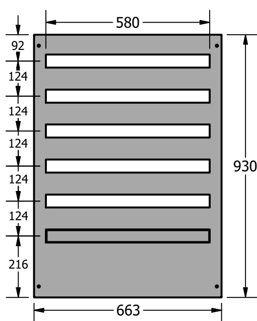
ΜΕΤΩΠΙΚΗ ΓΙΑ ΚΙΒΩΤΙΟ 70X100 6 ΣΕΙΡΩΝ
