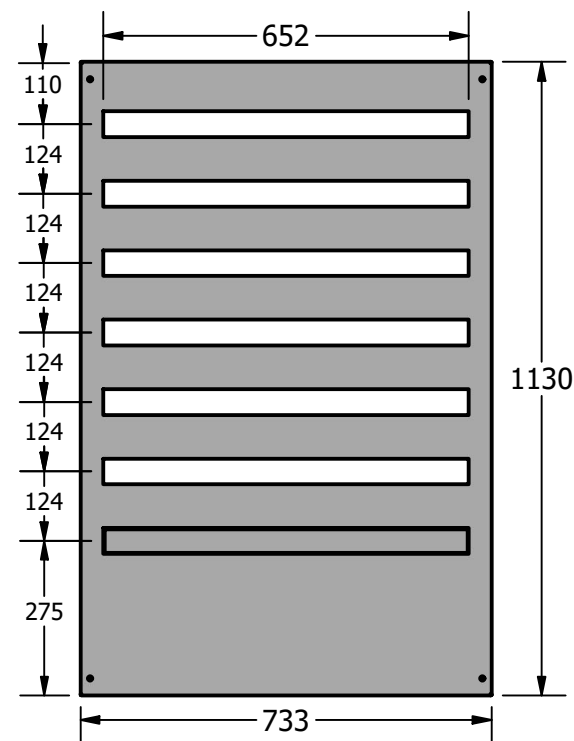
ΜΕΤΩΠΙΚΗ ΓΙΑ ΚΙΒΩΤΙΟ 80X120 7 ΣΕΙΡΩΝ
